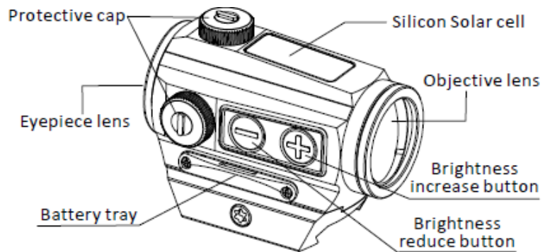
Fig1 PARALOW HS403C Red Dot Sight
